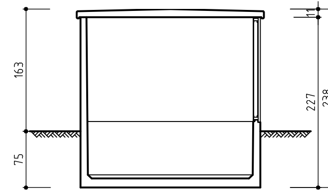
Schnitt A-A
