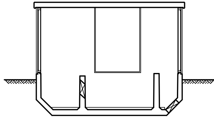
Schnitt B-B
